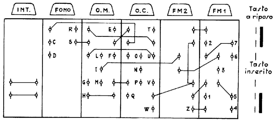
RADIORICEVITORE PANART Mod. « REFRAIN »
